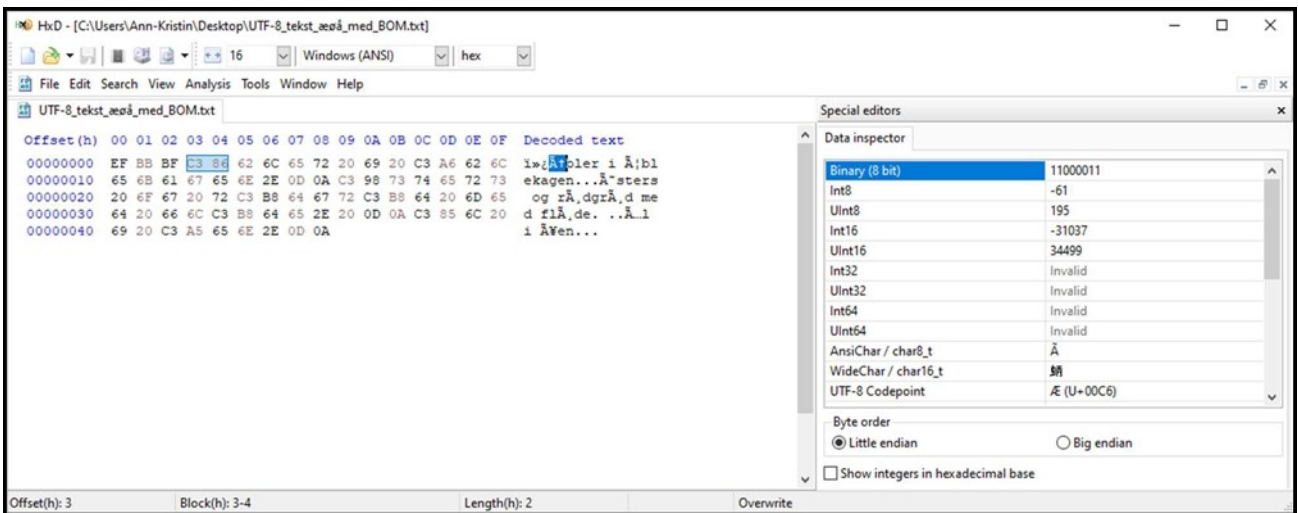
Figur 13 UTF-8 fil med Stort Æ (hexadecimale værdier: C3 86)
