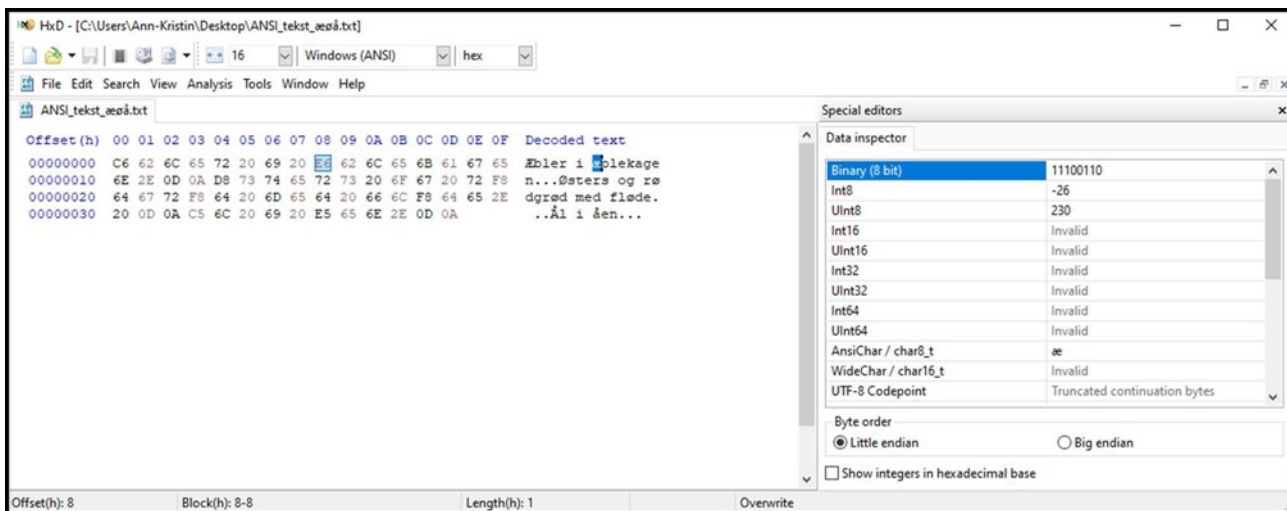
Figur 16 ANSI fil med lille æ (hexadecimale værdier: E6)
