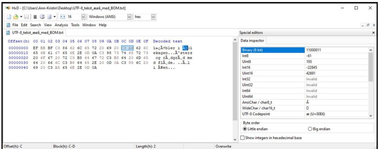
Figur 10 UTF-8 fil med lille æ (hexadecimale værdier: C3 A6)
