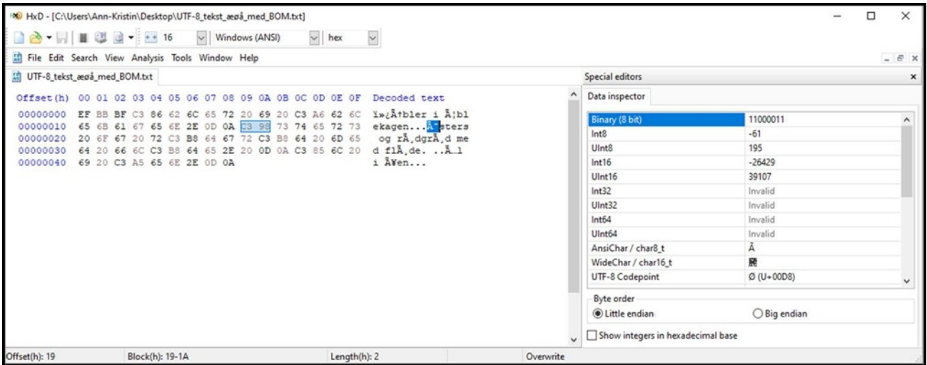
Figur 14 UTF-8 fil med Stort Ø (hexadecimale værdier: C3 98)
