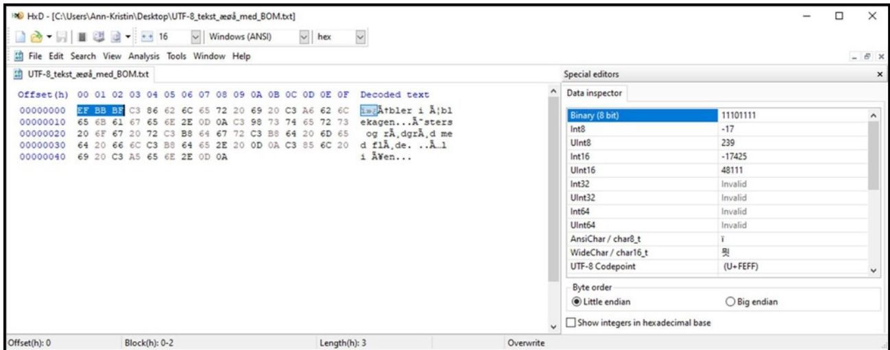
Figur 8 UTF-8 fil med BOM (hexadecimal værdier: EF BB BF)
