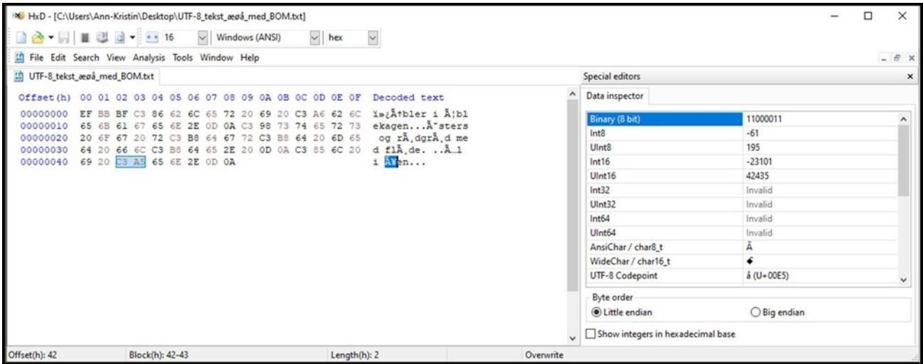
Figur 12 UTF-8 fil med lille å (hexadecimale værdier: C3 A5)
