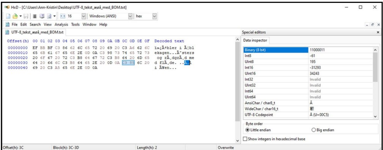
Figur 15 UTF-8 fil med Stort Å (hexadecimale værdier: C3 85)
