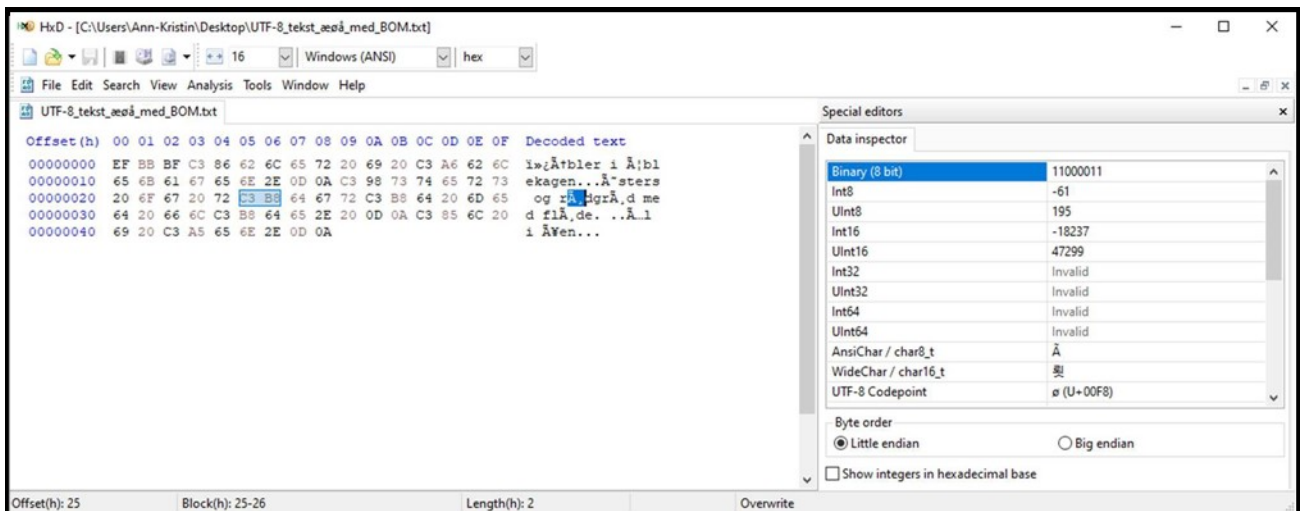
Figur 11 UTF-8 fil med lille ø (hexadecimale værdier: C3 B8)
