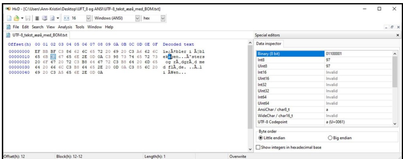
Figur 9 UTF-8 fil med lille a (hexadecimale værdi: 61)
